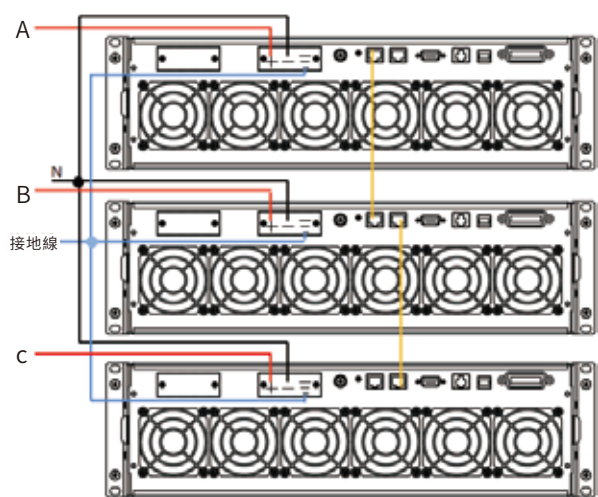
星形接法
