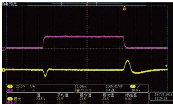
單機 IT6006B-500-40 500V 40A 6000W 設定電壓:100V 設定電流:28A 負載電流:30A
