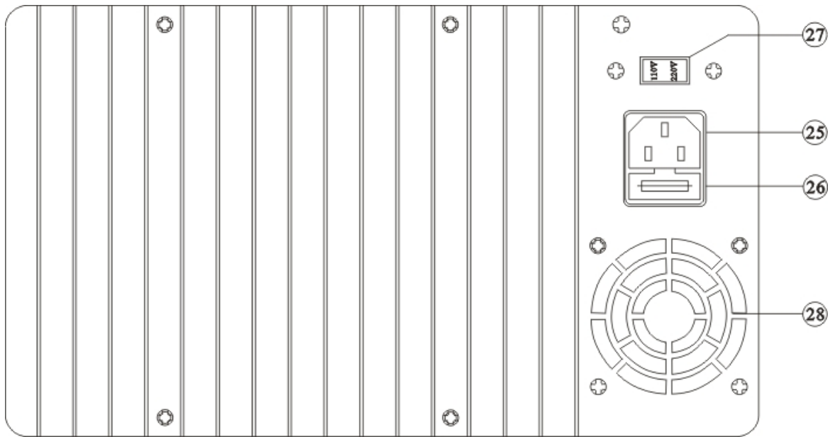
圖 4.2 後面板 (TP-30102/TP-60052)
