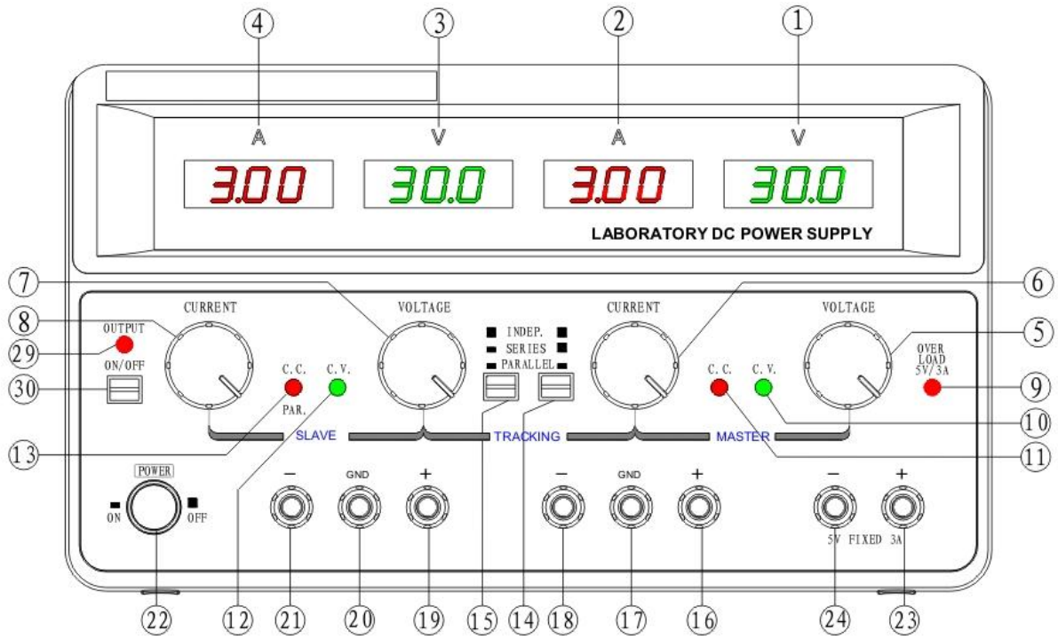
圖 3.1 前面板 (TP-2303TK/TP-2305TK)
