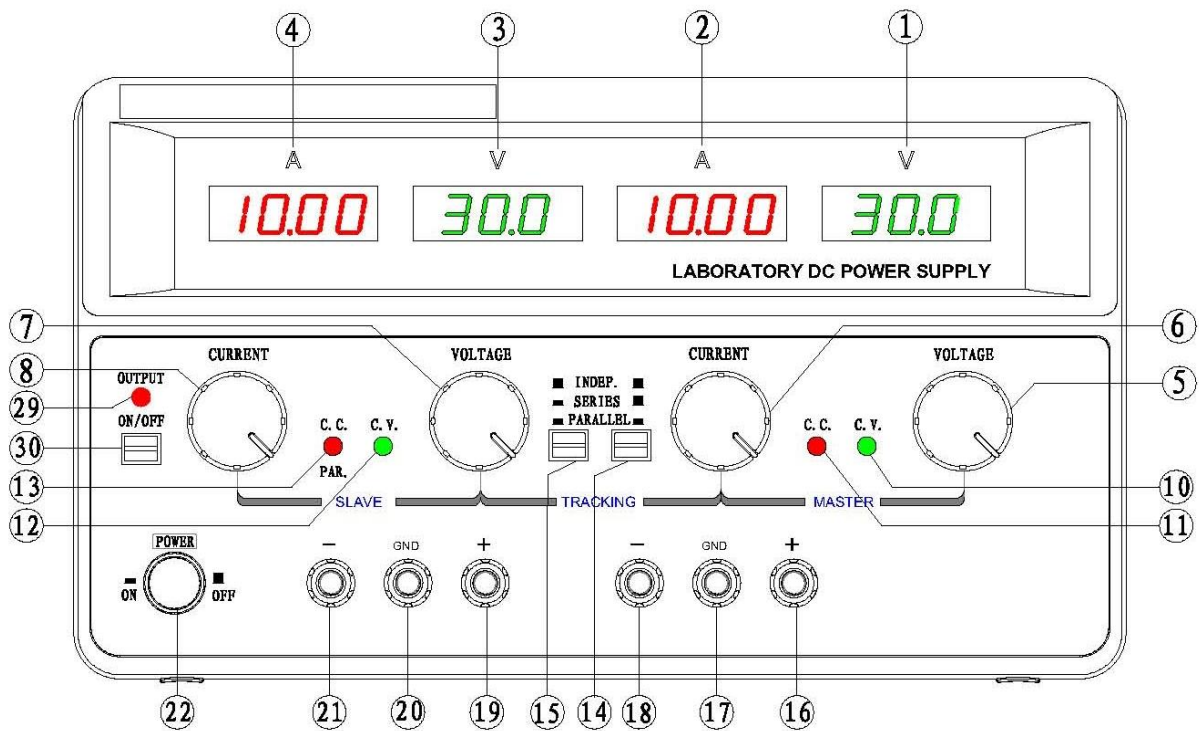
圖 4.1 前面板 (TP-30102/TP-60052)
