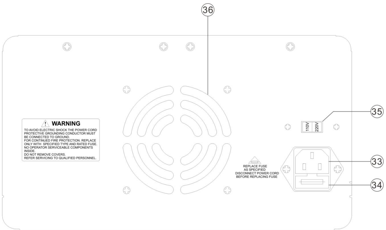
圖 3.2 後面板
